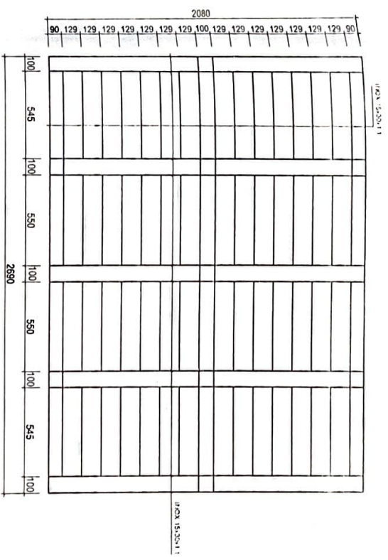
HOA SẮT CỬA S2 (3CK)
