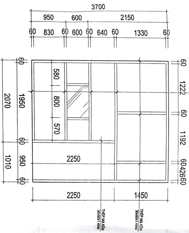
KHUNG ĐỠ VÁCH
