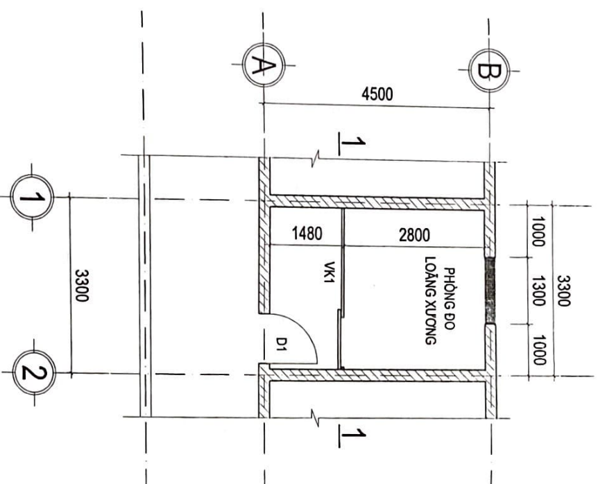
MẶT BẰNG CẢI TẠO
