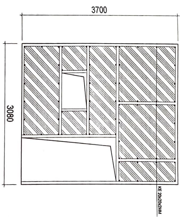
CHI TIẾT LỚP GIỮA VÁCH
