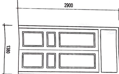
D3; 1 BÓ - PHÒNG HÀNH CHÍNH - CỬA GỖ, KHUÔN KÉP
