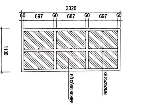
CT CẢNH CỬA LỚP GIỮA
