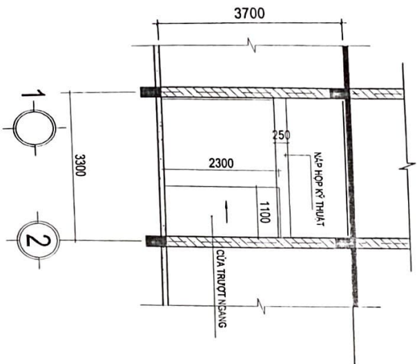
CHI TIẾT CỬA
