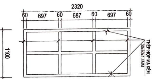
CT KHUNG CẢNH CỬA
