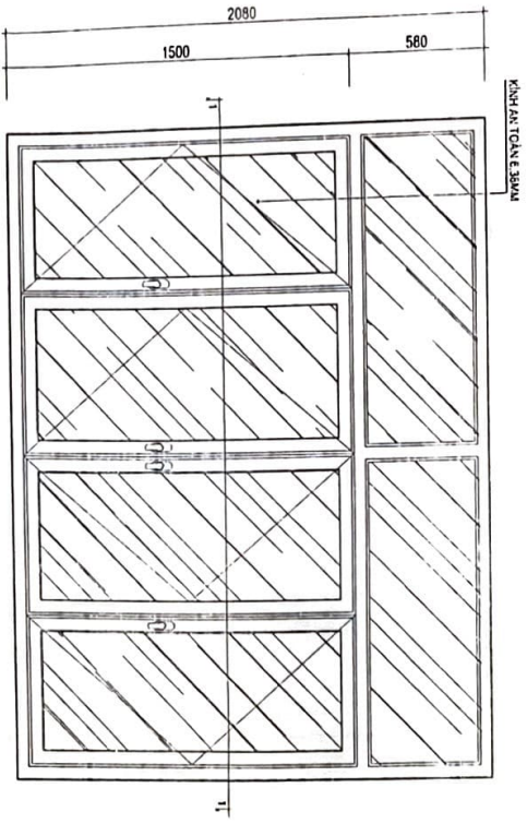
MẶT ĐƯNG CỬA S2
