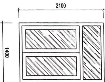
S1; 4 BÓ - CỬA GỖ, KHUÔN KÉP
